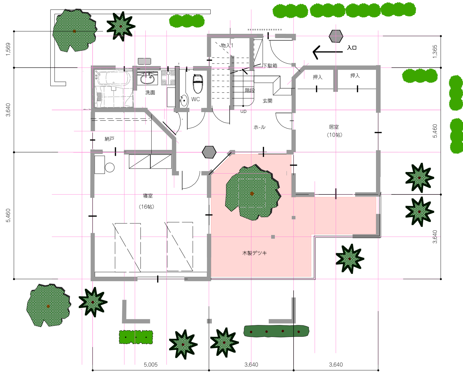
1階平面図 1/100
