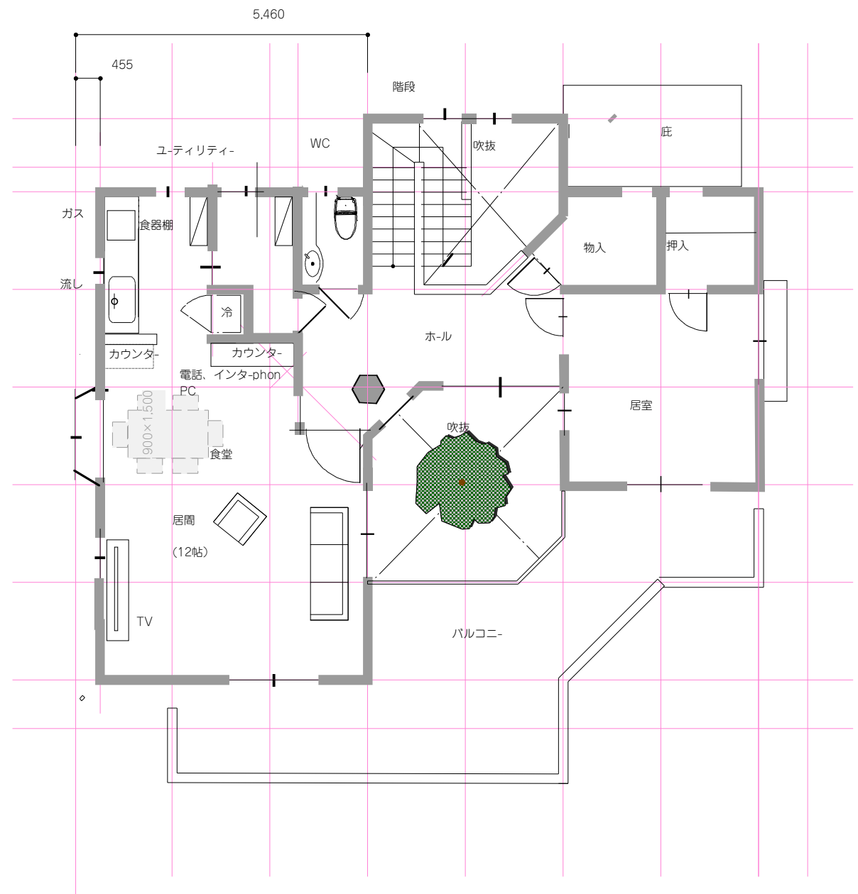
2階平面図 1/100
