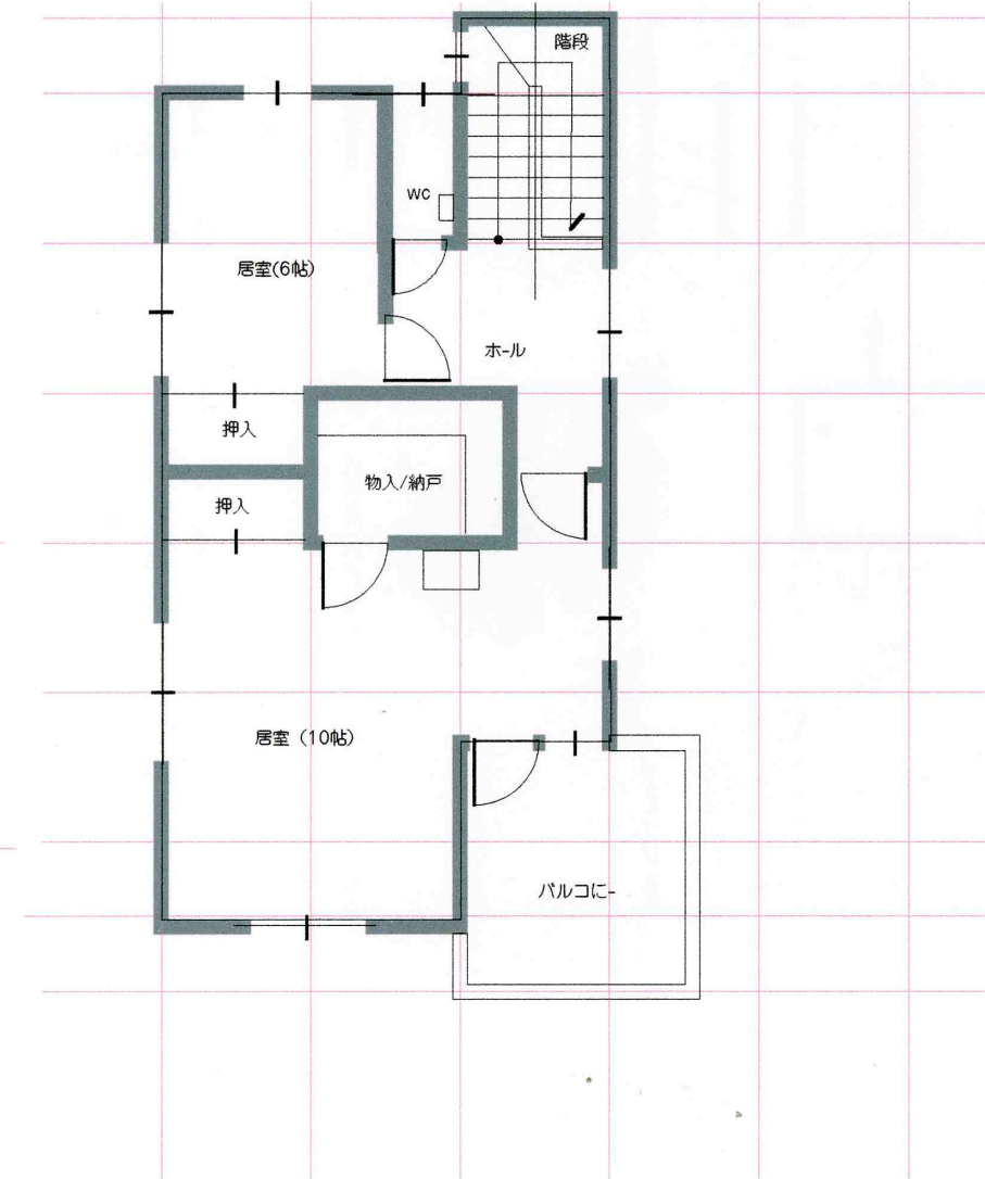
2階平面図 1/100
