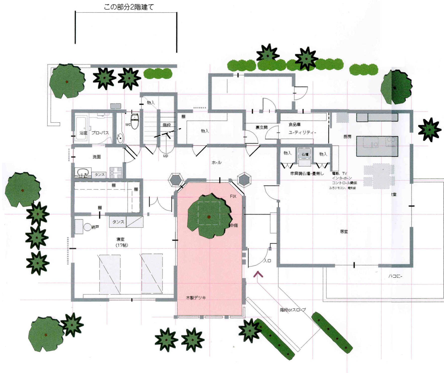
1階平面図 1/100
